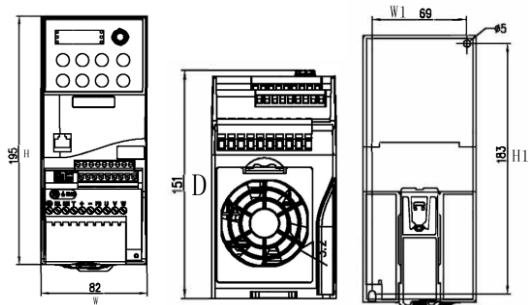
图2-3 SC300 系列变频器标准外形尺寸(适用于 0.7~4kW 机型)
