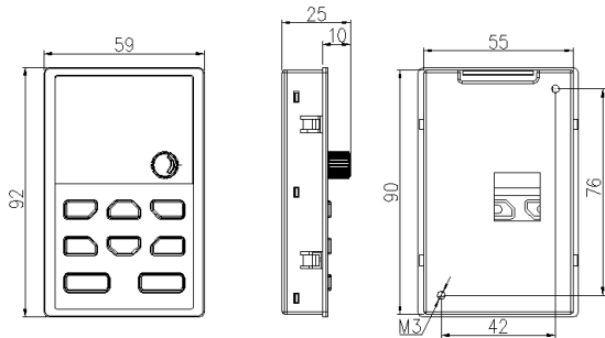
图2-4 键盘安装开孔尺寸 55*90（mm）
