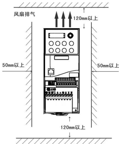
图3-1 变频器安装间隔距离
