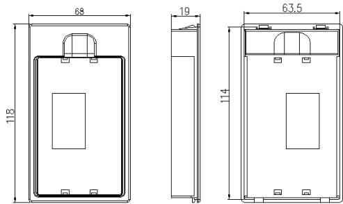
图2-5 键盘托安装开孔尺寸 63.5*114（mm）
