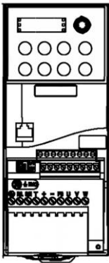
图3-6 0.75~4.0kW 主回路端子
