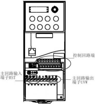
图3-5 主回路端子位置示意图
