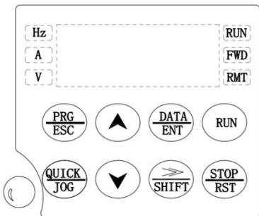
LED 键盘显示单元示意图
