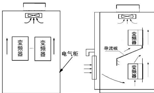
(a) 2-2 多台变频器的安装 (b)
