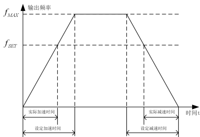
加减速时间示意图
