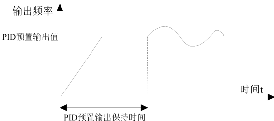
PID 预置输出示意图
