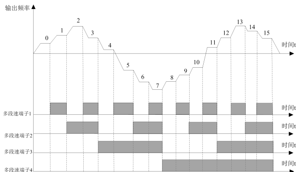
多段速运行示意图
