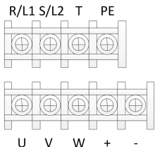
0.75~2.2KW 机型主回路端子
