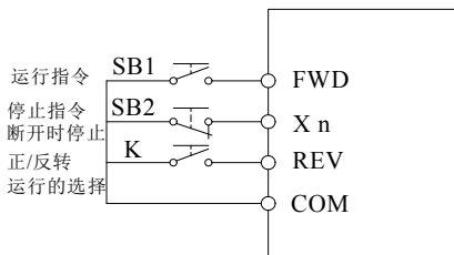
3 线制顺序控制模式 2
