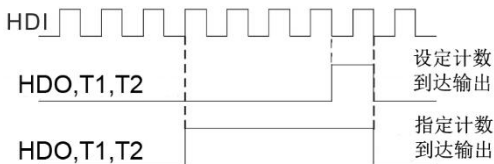
设定计数值和指定计数值示意图
