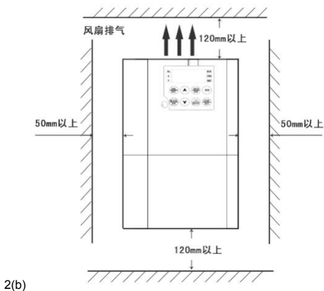
2-1 变频器安装间隔距离
