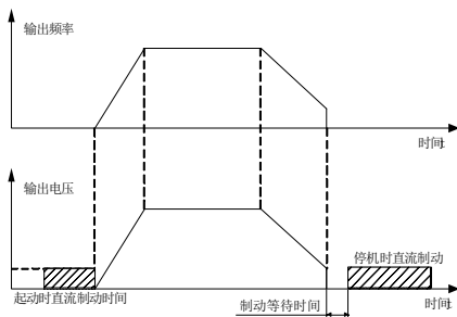
直流制动示意图
