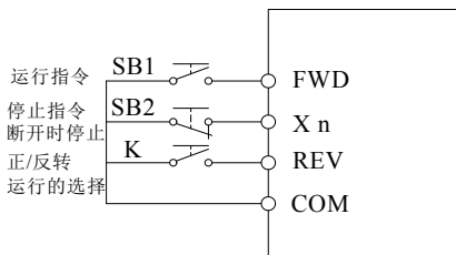
3 线制顺序控制模式 1
