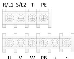
4~11KW 机型主回路端子
